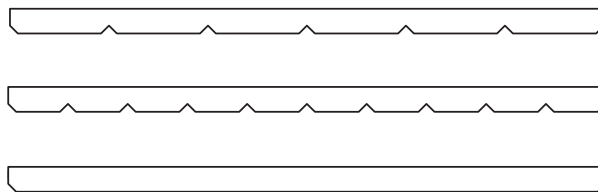
Doorsneden van Troldtekt v-line 1way 6, v-line 1way 10 en v-line 1way blank. Afmetingen paneel: 25 x 600 x 1200 mm.
