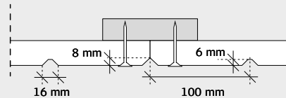
DWARSDOORSNEDE Troldtekt® wall deco/v-line 6 100 mm afstand tussen de groeven
