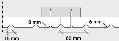
DWARSDOORSNEDE Troldtekt® wall deco/v-line 10 60 mm afstand tussen de groeven
