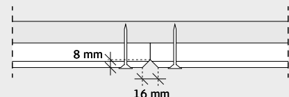
LENGTEDOORSNEDE Troldtekt® wall deco/ v-line 6 en v-line 10 100 mm afstand tussen de groeven
