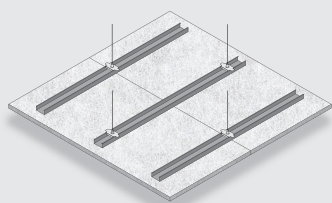
Fig. 1 Troldtekt Elements zwevend plafond gemonteerd
